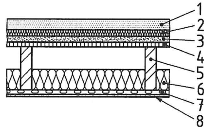
Bild D.4 — Deckenkonstruktion der Wohnungstrenndecke
